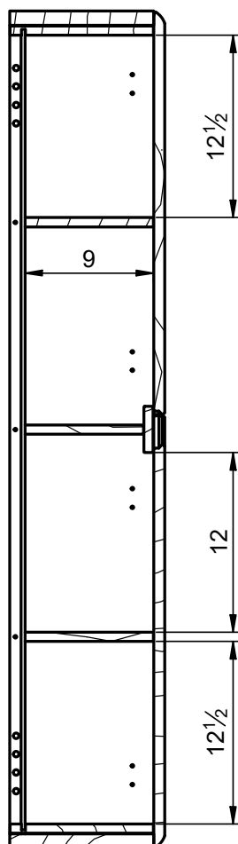
B-B ( 1:10 )
