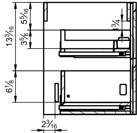
B-B ( 1 : 10 )
