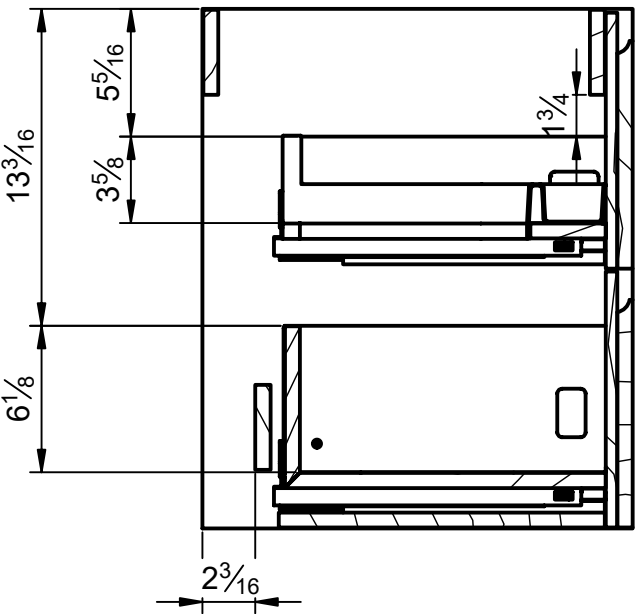
B-B ( 1 : 8 )
