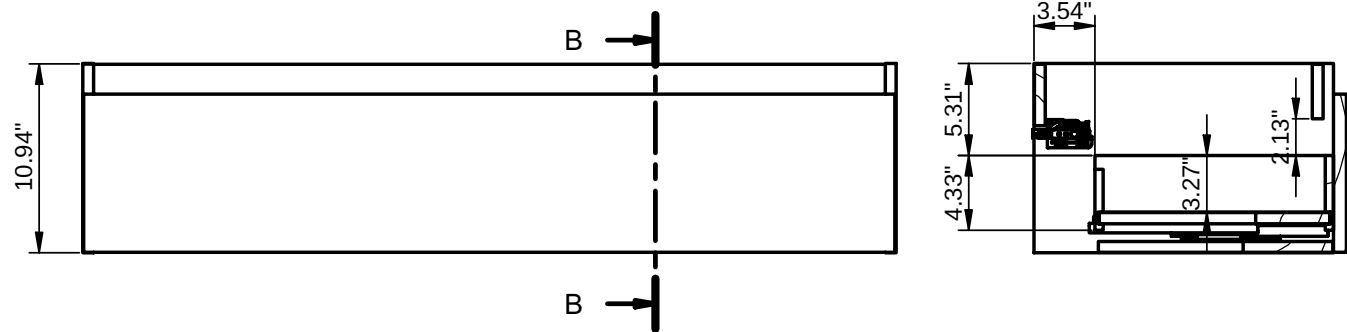
B-B ( 1 : 10 )
