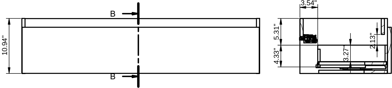
B-B ( 1 : 10 )
