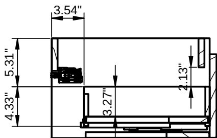
B-B ( 1 : 10 )
