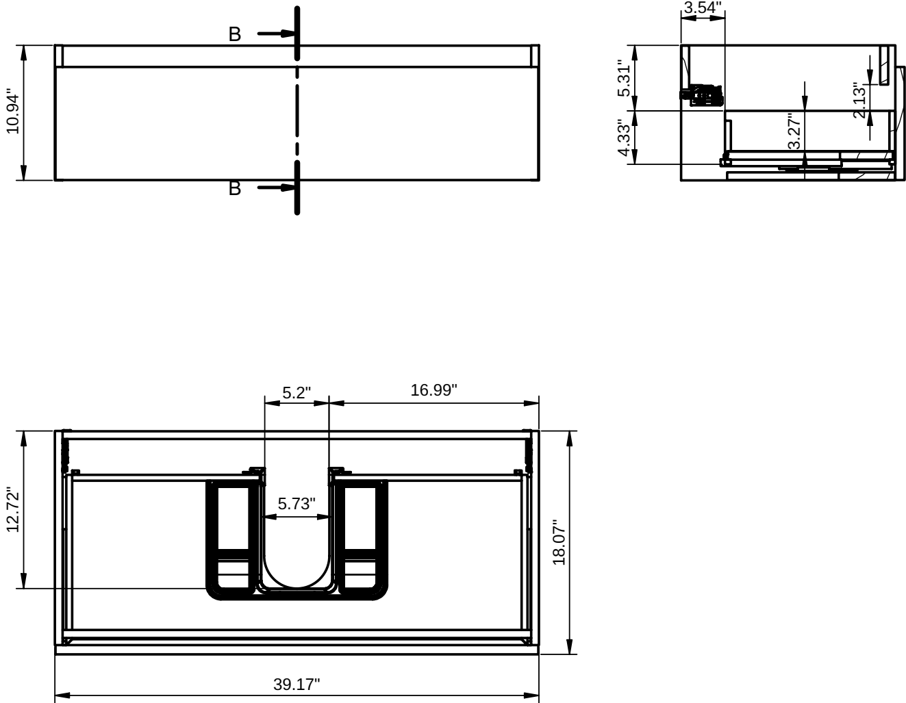
B-B ( 1 : 10 )
