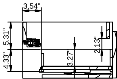
B-B ( 1 : 10 )
