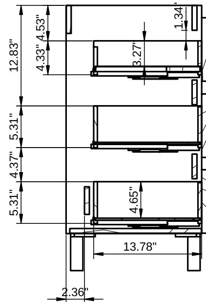
B-B ( 1 : 10 )
