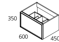
Mueble ALTAI 1C. 60 ALTAI vanity 60 1Dwr. 60 x 45 x 35 cm
